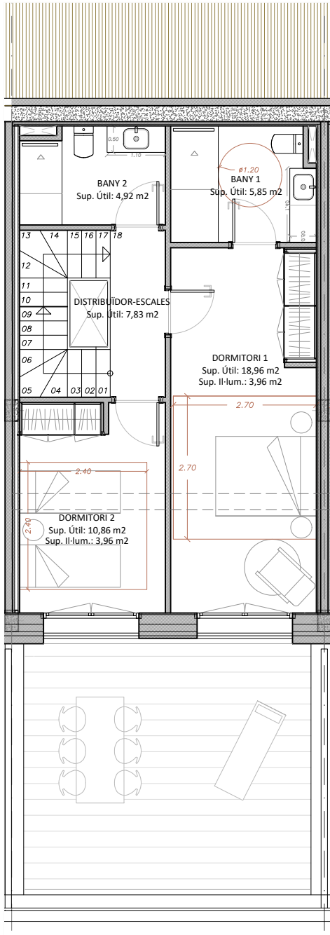
PLANTA PRIMERA
